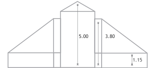
Hall Sala de Cámara. Sección E- E'
